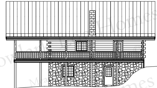
RIGHT ELEVATION
